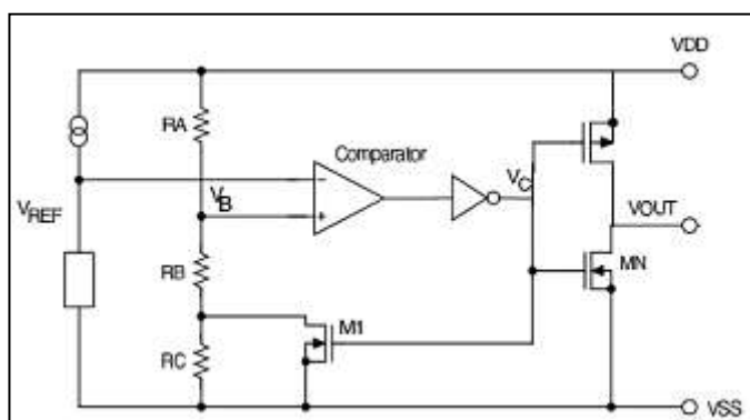
Fig.1 CMOS output voltage detector (ME2807)
